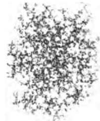
Fig. 8. Nuclein aus Hefe, 3-proc. in 0,5 KOH, mit FLEMMING'scher Lösung gefällt; rein-gerinnelig. (Vergr. 1500.)
